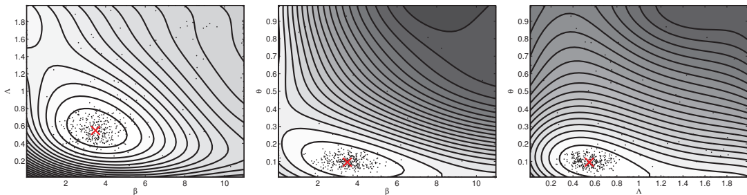
(d) 500 data points, \hat{\theta}_J^{(500)} = (3.50, 0.55, 0.10)
